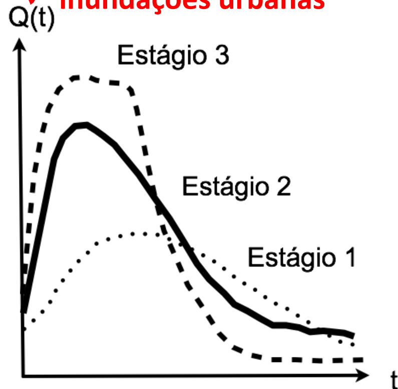
Hidrograma Ponto de Controle A
